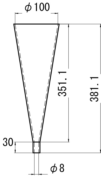
約1000ml J Aコーン (土木学会規準)
