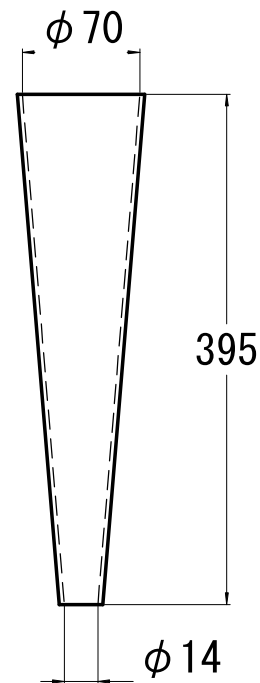
約628ml Jコーン14 (道路公団規格)
