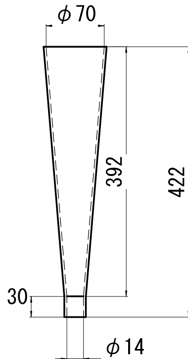
約627ml J Pコーン (土木学会規準)
